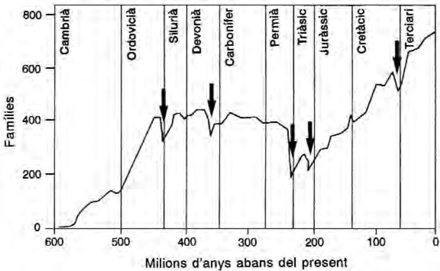
FIGURA 6. En el passat geològic s'han produït diverses crisis de biodiversitat, ocasionades per catàstrofes naturals d'origen incert. En el gràfic es destaquen les cinc més importants, indicades amb fletxes. La biodiversitat s'ha evaluat amb les dades de famílies d'organismes marins. El gràfic és una versió lleugerament modificada del que presentà E. O. Wilson el 1992.
